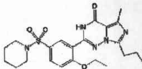
プソイドバルデナフィル(pseudovardenafil)
