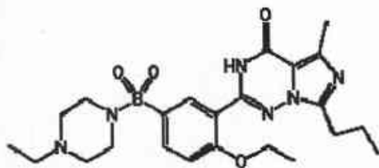
バルデナフィル(vardenafil)
