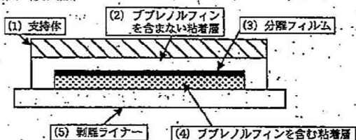
外形 断面図 (模式図)
