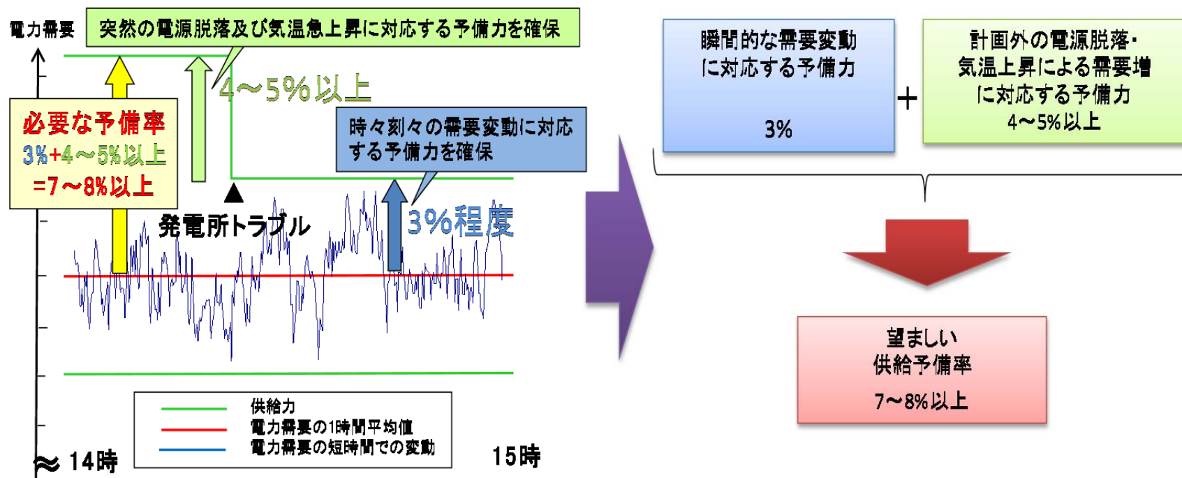
図3-1 供給予備率の考え方
