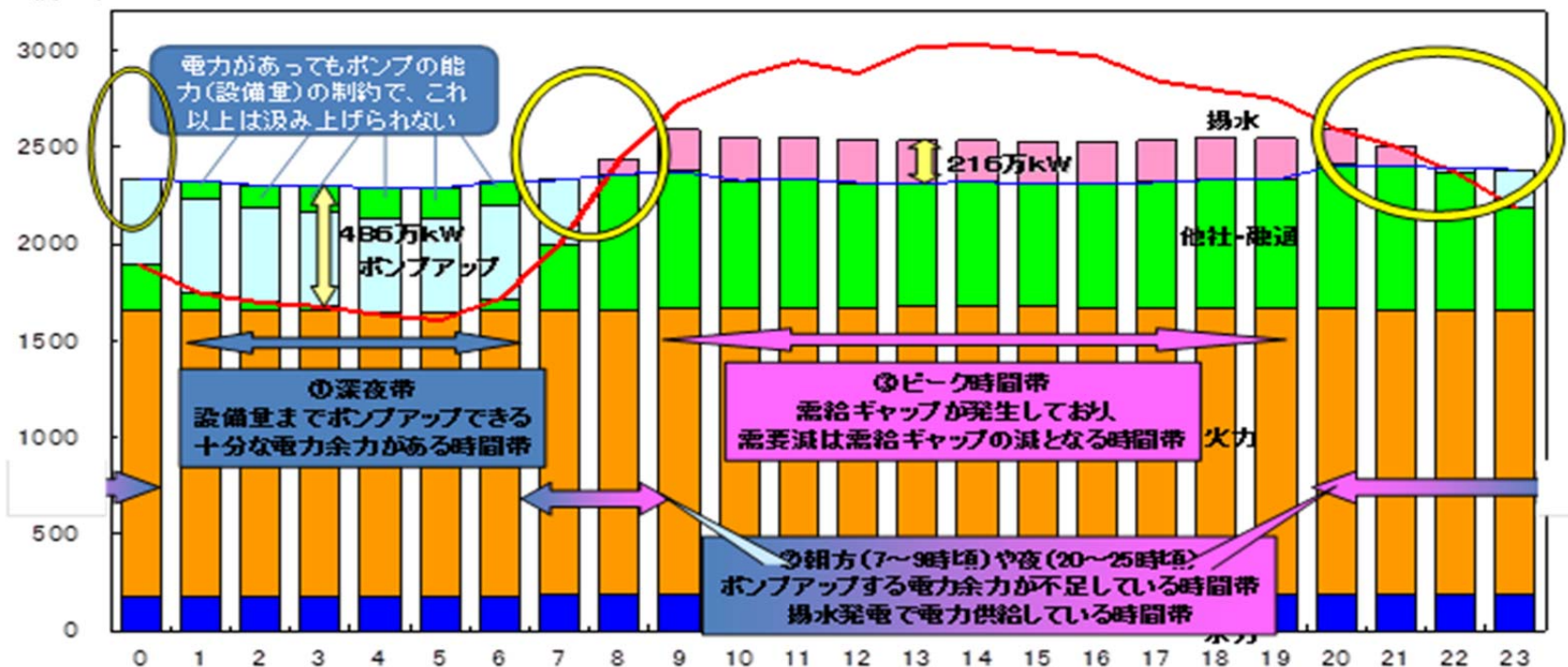
図5-1 揚水の供給力改善に効果がある節電効果の時間帯(関西電力の例)
