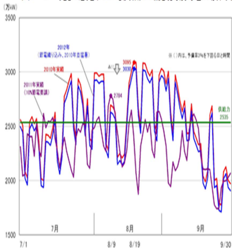
図5-2 今夏で想定している供給力と需要実績等を比較し、後者が上回ると予想される日数、時間(関西電力)
