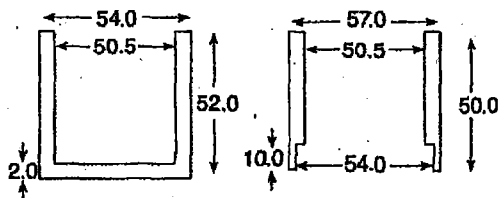
図 3.01-2 測定用容器 (左) と補助円筒 (右) 単位: mm
